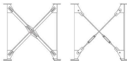
アングルブレース
