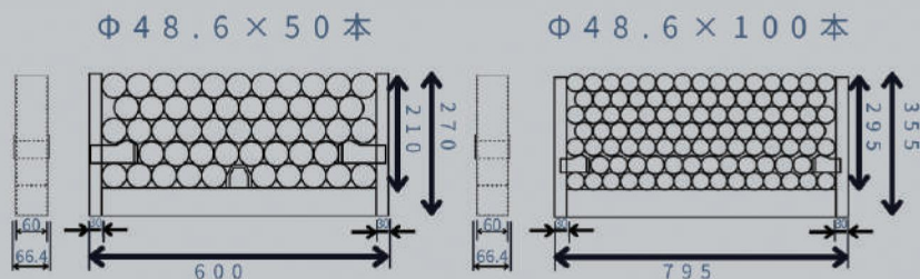
■寸法図
